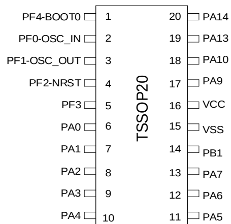
图 3-10 TSSOP20 Pinout3 PY32F030F3xP
